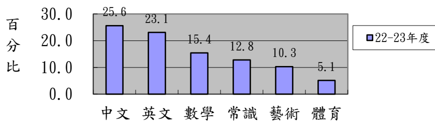
小四至小六授課時間分佈
