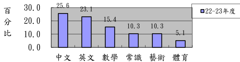
小一至小三授課時間分佈
